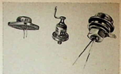
Bild 3. Leistungstransistoren OC 30 und OC 16 der Valvo GmbH; in der Mitte die Leistungsdiode OA 31
