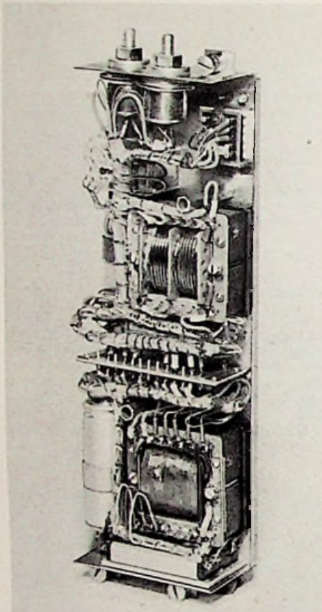
Bild 2. Stromversorgung für Sender und Empfänger des Philips-Lotsen-Funksprechgerätes „Portofon“ mit zwei Transistoren als Schalter (DC-Converter)
