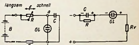
Links: Bild 1. Ladewiderstand R und Ladekondensator C der Glimmröhrenkippschaltung liegen in Serie. Mit R kann die Kippfrequenz f eingestellt werden
