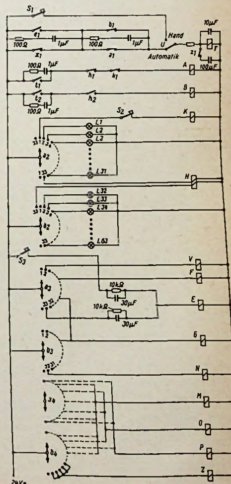
Bild 1. Steuerteil A des Kontrollgerätes für maximal 63 Meßstellen. Die Bezeichnungen sind in allen Zeichnungen einheitlich:
