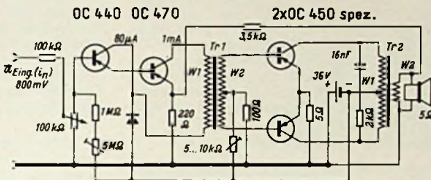
Bild 8. Schaltung eines Niederfrequenzverstärkers mit Intermetall-Siliziumtransistoren für hohe Umgebungstemperaturen.
