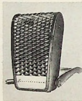
Bild 3. Super-Kardloid-Mikrofon MD 403 vom Labor W
