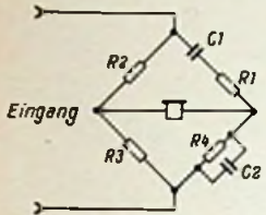
Bild 1. Wienbrücke zur Bestimmung von Tonfrequenzen
