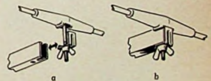
Bild 4. Befestigung der Elemente (Direktor 1 und Reflektor) an den Enden des Abstandsrohres einer Band-III-Antenne von Kathrein
