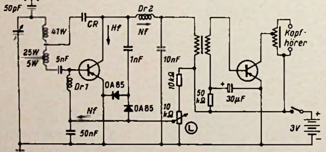
Bild 1. Schaltung des Transistor-Reflexempfängers. Alle Widerstände sind vom 0,5-W-Typ, die Kondensatoren für 10 V Arbeitsspannung
