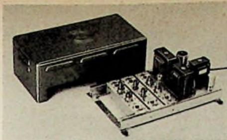
Bild 1. Antennenvorverstärker bestückt mit drei Streifen (UKW, Fernsehkanal 3 und 8) und gemeinsamen Netzteil von Wisi (Modell 188 VN)
