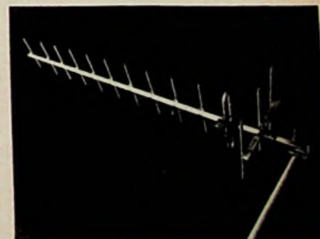
Bild 5. Antenne für Band IV mit Dipol, zehn Direktoren und Reflektorwand (Wisi Modell 910)
