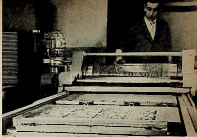
Bild 1. Mit dieser Offset-Presse werden die Schaltungen auf die kupferkaschierten Platten mit einer ätzfesten und lötfähigen Farbe gedruckt
