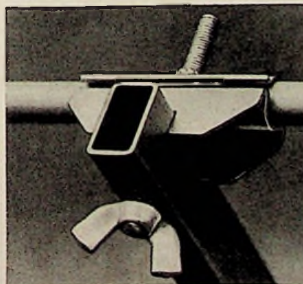
Bild 3. Prinzip der gefalteten Antennenstäbe bei Fuba; oben: die beiden Stabhälften werden durch eine Klammer am Tragerohr gehalten, unten: Stäbe fertig montiert
