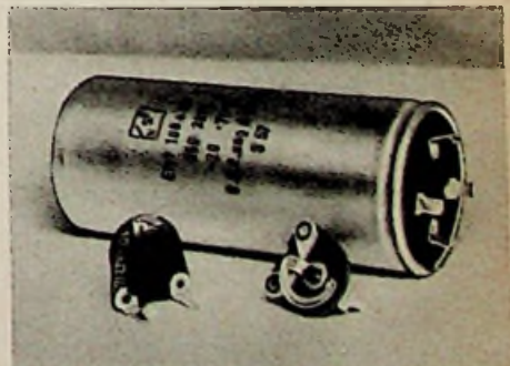
Bauelemente mit snap-in-Anschlüssen für das genormte Rastermaß gedruckter Schaltungen (Doppel-Elektrolytkondensator und Trimpotentiometer von NSF)
