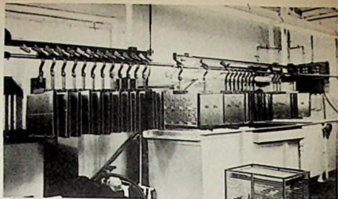
Bild 6. Vollautomatische Ätzanlage. Die mit ätzfester und lötfähiger Farbe bedruckten Platten werden geätzt, gespült und gewässert. Der letzte Arbeitsvorgang in dieser Etappe ist die Trocknung
