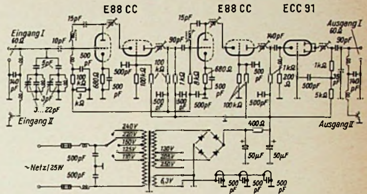
Bild 1. Antennenvorverstärker bestückt mit drei Streifen (UKW, Fernsehkanal 3 und 8) und gemeinsamen Netzteil von Wisi (Modell 188 VN)
