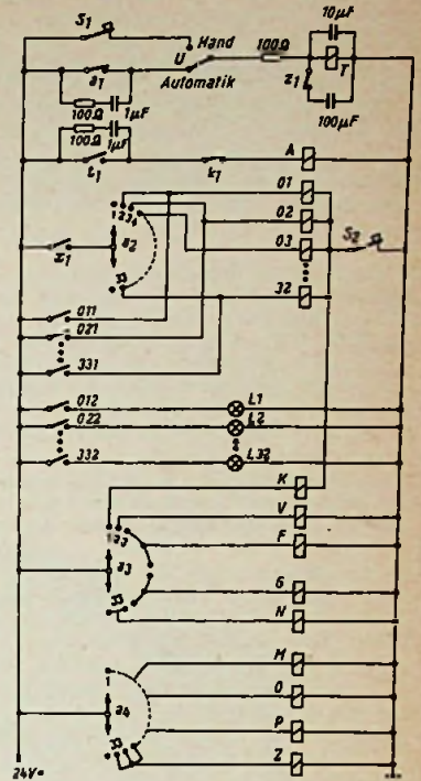
Bild 6. Vereinfachtes Steuerteil B für maximal 32 Meßstellen
