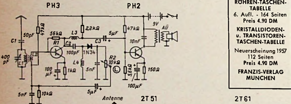
Bild 1. Schaltung des Transistor-Reflexempfängers. Alle Widerstände sind vom 0,5-W-Typ, die Kondensatoren für 10 V Arbeitsspannung
