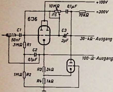
Bild 1. Schaltung eines Tastkopfs mit fast unendlich großer Eingangsimpedanz
