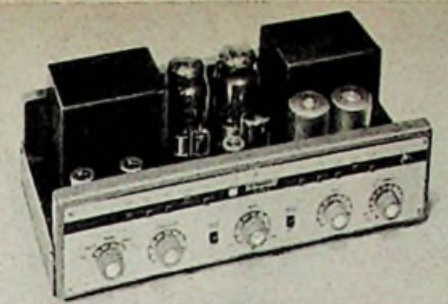
Bild 8. „Telewatt Ultra“, ein 40-W-Hi-Fi-Verstärker (Klein & Hummel)
