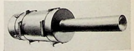
Bild 3. Wasser- und luftgekühlte Industrie-Fernsehkamera mit nur 5 mm Sondenöffnung zur Beobachtung von Feuerräumen und Ofen mit Innentemperaturen bis zu + 1800^\circ C (Siemens)
