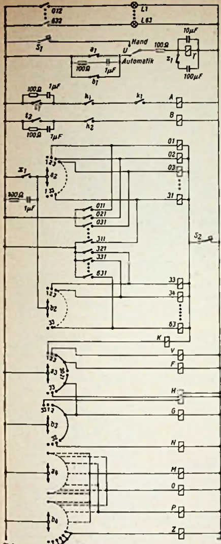
Bild 4. Steuerteil B des Kontrollgerätes für maximal 63 Meßstellen
