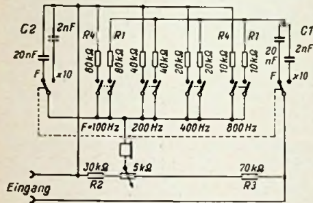
Bild 2. Schaltung eines Gerätes zur Bestimmung von Tonfrequenzen im Hörbereich
