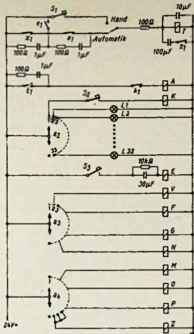
Bild 5. Vereinfachtes Steuerteil A für maximal 32 Meßstellen
