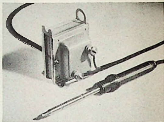
Bild 1. Ein nur 100 Gramm schwerer, in sechs Sekunden anheizender LötKolben mit der Leistung eines 150-W-Kolbens ("Superspeed Soldering Iron")
