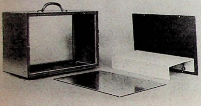
Oben: Bild 1. Bestandteile für ein selbstgebautes Gehäuse. Sehr zweckmäßig erweisen sich Vierkant-Aluminiumstangen für die Rahmen innerhalb der Zarge und U-Profil für das Chassis
