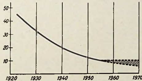
Bild 2. Die durchschnittliche Herstellzeit eines Mittelklassen-Rundfunkempfängers ab 1923. Die links angegebenen Zahlen entsprechen den Arbeitsstunden je Gerät. Ohne Übergang zur neuen Technik läßt sich die Arbeitszeit vermutlich kaum mehr weiter herabsetzen (obere gestrichelte Kurve)
