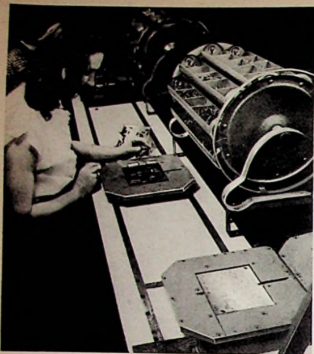
Links: Bild 5. Bestückungsplatz für gedruckte Schaltungen. Die Arbeiterinnen erlangen nach kurzer Zeit eine solche Gewandtheit, daß je Platz eine große Anzahl verschiedener Teile fehlerfrei eingesetzt werden kann, daher die großen Vorrattrommeln
